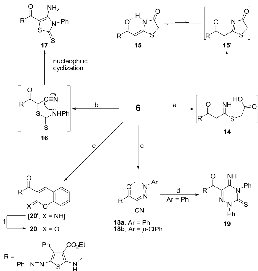
Scheme 3. Reagents and conditions: (a) HSCH 2 CO 2 H, AcOH, reflux; (b) S 8 , PhNCS, EtOH, Et 3 N, reflux; (c) ArN 2 Cl, EtOH, AcONa, 0–5 °C; (d) PhNCS, EtOH, Et 3 N, reflux; (e) o -HOPhCHO, EtOH, piperidine, reflux; (f) EtOH, HCl, reflux.
